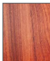
64 Mahagón červený
